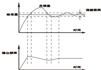
偏差极限与输出频率的对应关系
